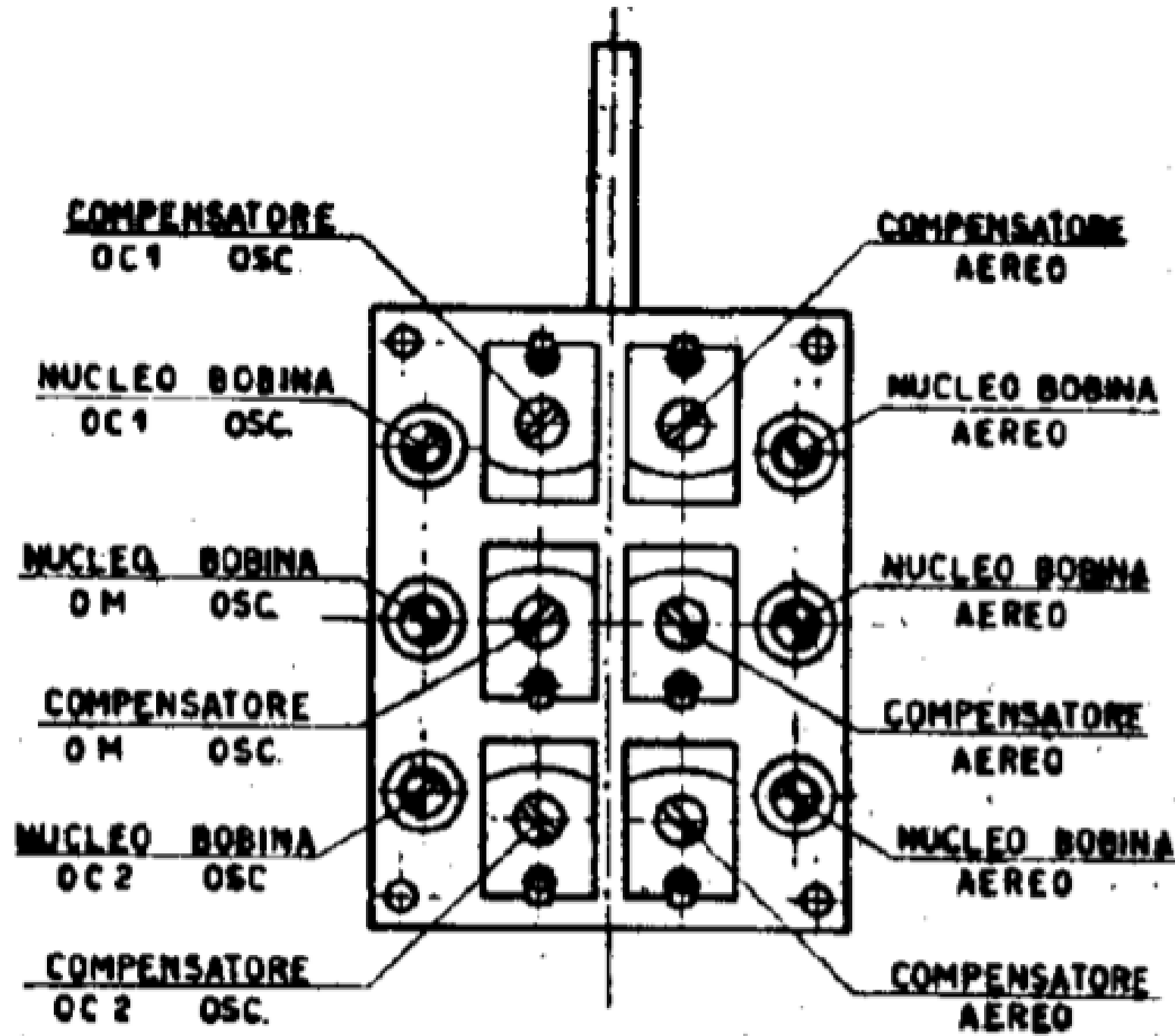
Il piano dei compensatori del Safer modd. « 538/A » « 538/B » « 538/RF » « 5310 »
